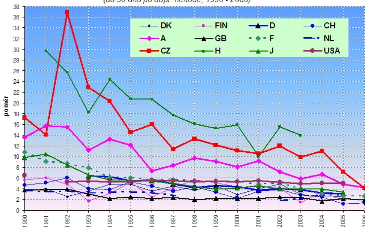
Graf 1: Usmrcení na dálnicích na 10exp9 vozidlokm (do 30 dnů po dopr. nehodě, 1990 - 2006)
