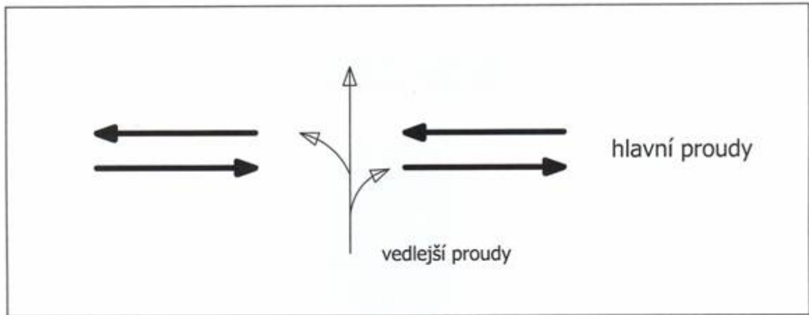
Obr.1 Schéma „volné křižovatky“ pro vedlejší proudy
