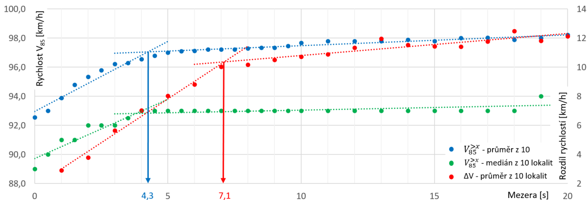
obr. 03. Pražská hodnota ovlivnění řidičů dle průběhu a z deseti lokalit silnice I. třídy
