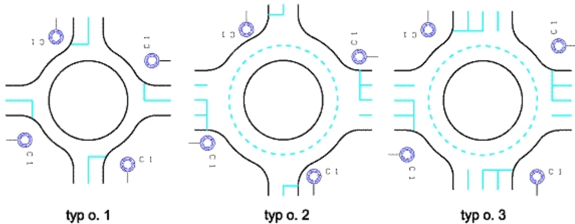
Dispoziční uspořádání typů okružních křižovatek
