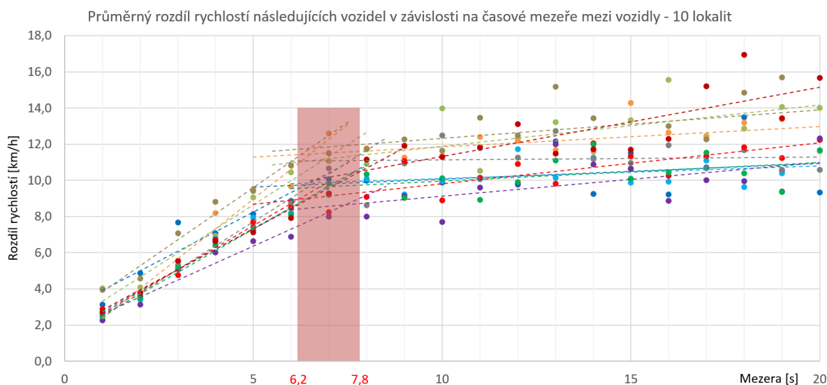
obr. 02. Prahou hodnota ovlivnění řidičů dle průměrného rozdílu rychlosti po sobě jedoucích vozidel
