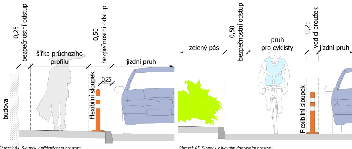
Obrázek 04. Sloupek v přidruženém prostoru
