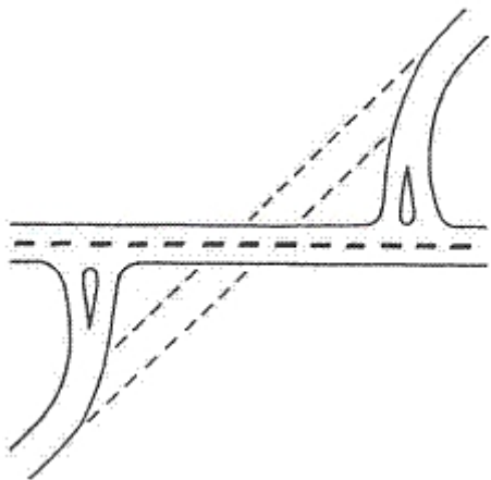
Obr. 21: Princip náhrady průsečné křižovatky s nevhodným úhlem křížení dvojitou stykových křižovatek
