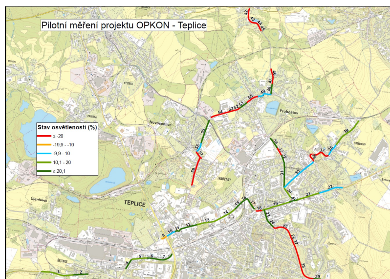
Mapa měření osvětlenosti komunikací Systémem MOMOK®
