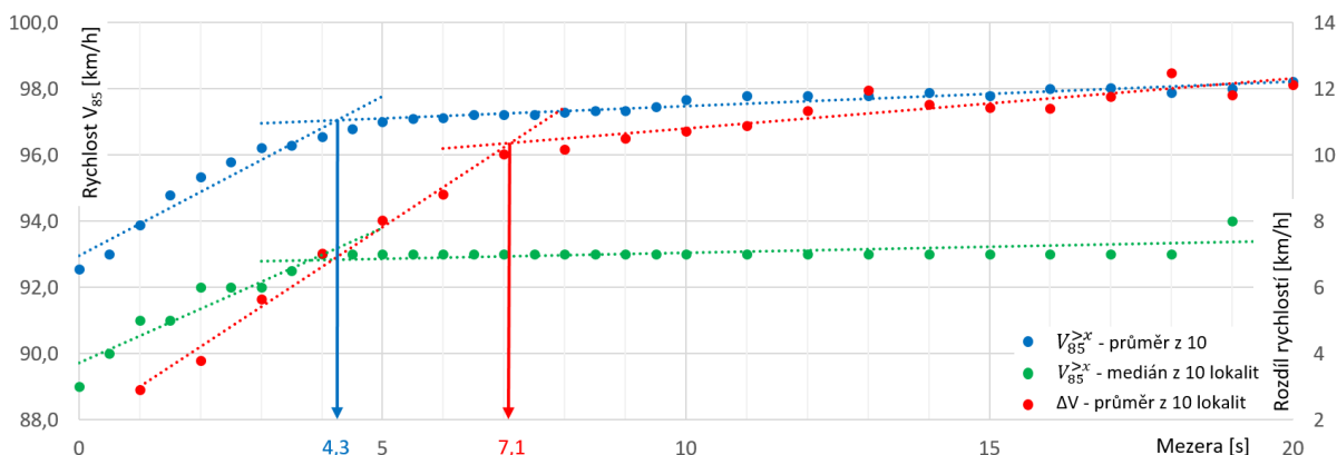
obr. 03. Práhová hodnota ovlivnění řidičů dle průběhu a z deseti lokalit silnice I. třídy
