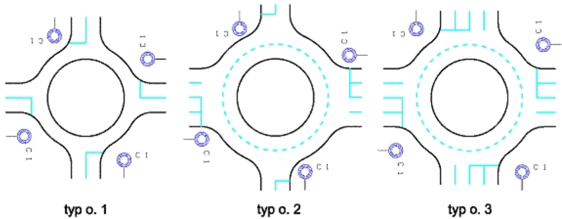
Dispoziční uspořádaní typů okružních křižovatek
