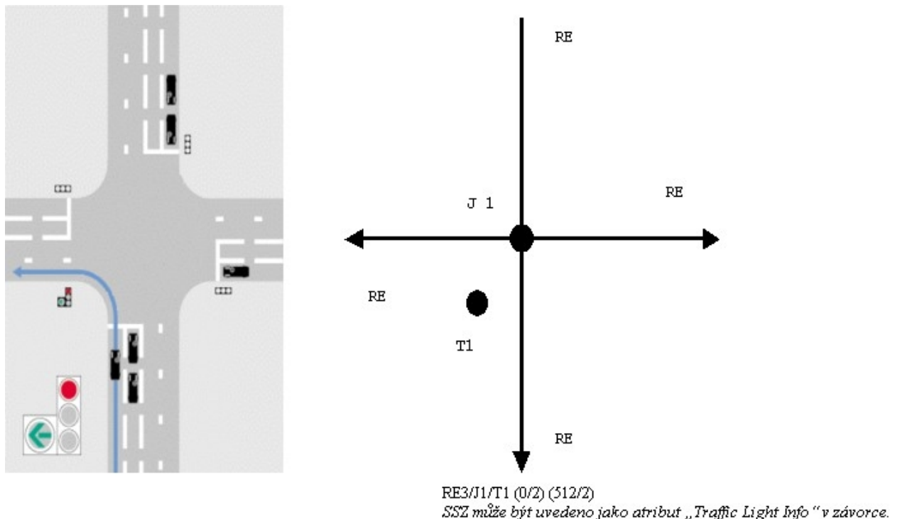
Obr. 5: Příklad řízení dopravy pomocí SSZ
