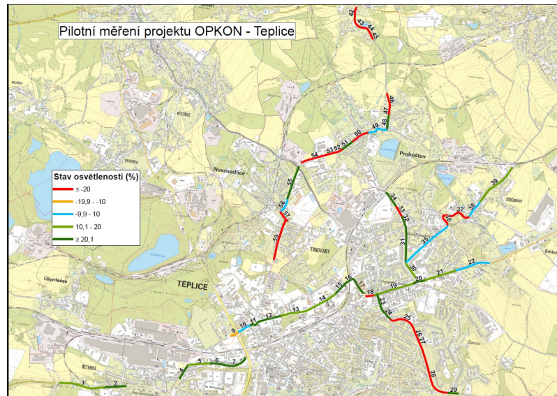
Mapa měření osvětlenosti komunikací Systémem MOMOK®
