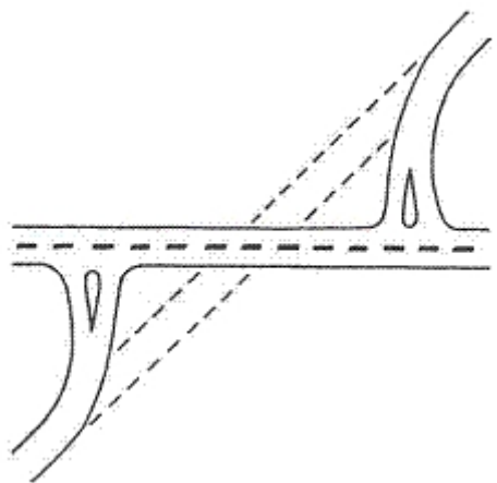
Obr. 21: Princip náhrady průsečné křižovatky s nevhodným úhlem křížení dvojitou stykových křižovatek
