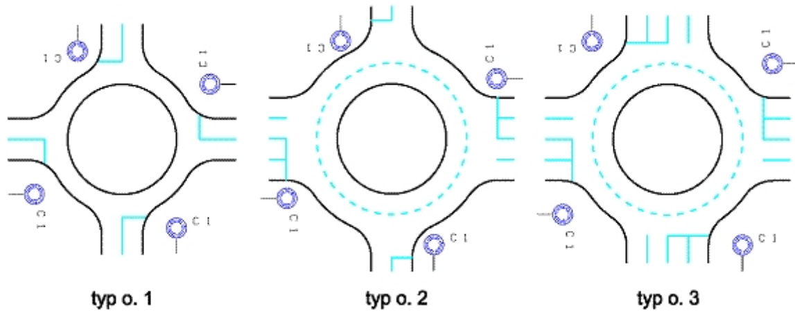
Dispoziční uspořádaní typů okružních křižovatek
