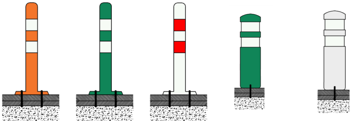
Obrázek 04. Směrové sloupky zelené kulaté - Baliseta
