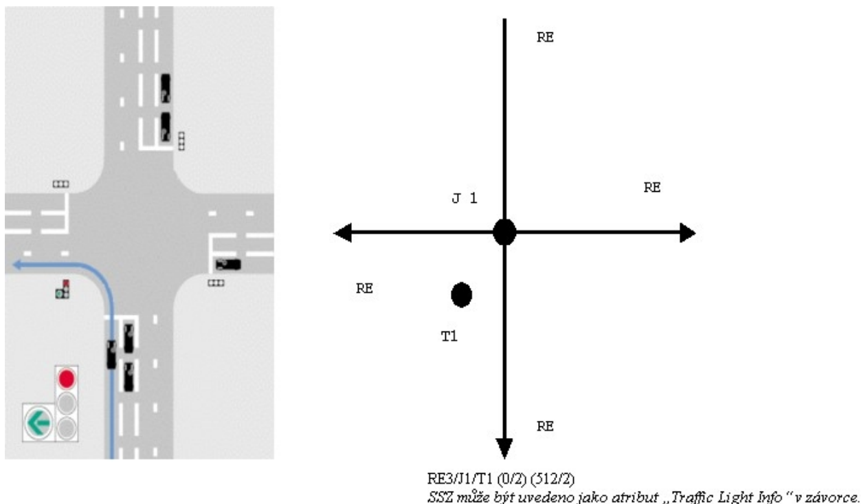
Obr. 5: Příklad řízení dopravy pomocí SSZ
