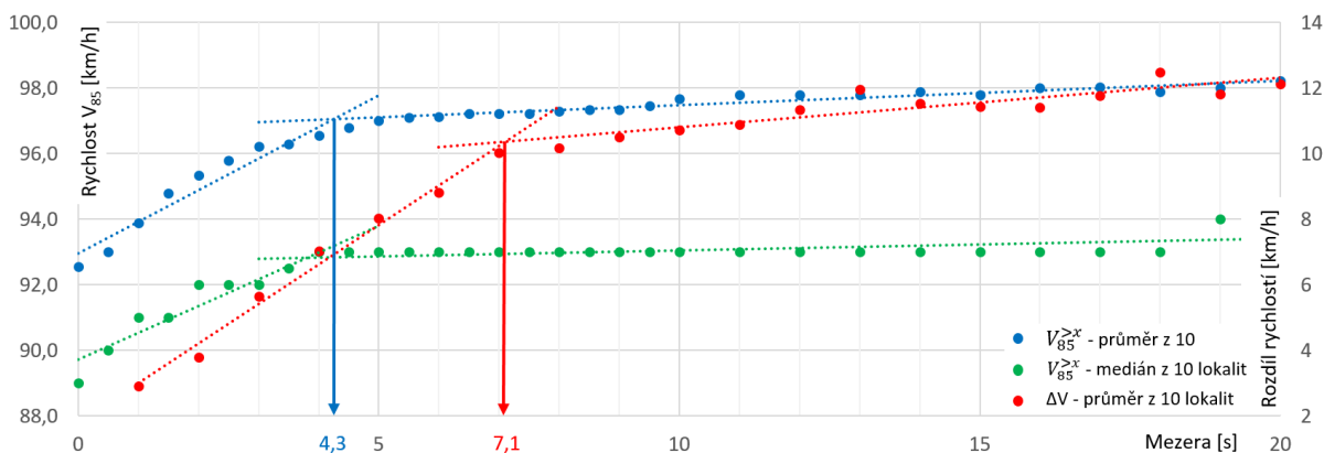
obr. 03. Prahavá hodnota ovlivnění řidičů dle průběhu a z deseti lokalit silnice I. třídy
