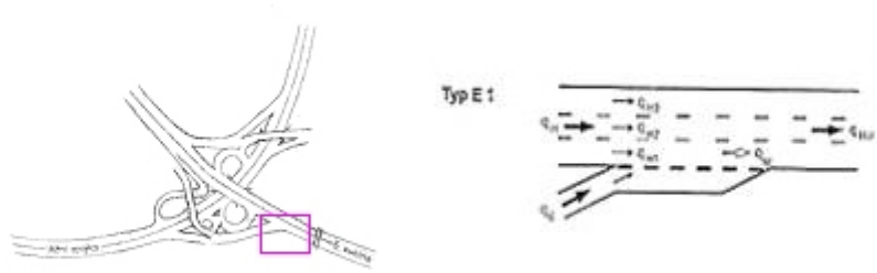
obr. č. 2 poloha a základní schéma připojení
