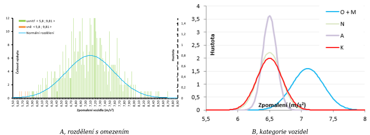
obr. 04 Modelované zpomalení vozidel pro brždění
